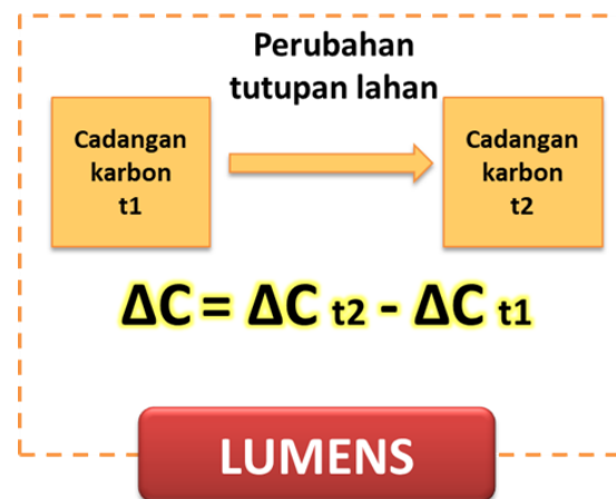
Gambar 8: Pendugaan perhitungan dinamika cadangan karbon
